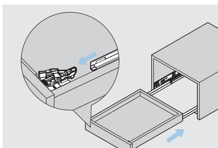
Apole o fundo da gaveta sobre a corrediça e, em seguida, empurre a gaveta para dentro do móvel.
