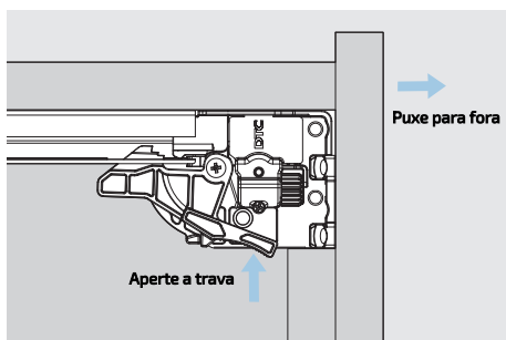
Para remover, aperte a trava e puxe a gaveta para fora.
